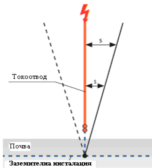
Фиг. 18. Потенциална разлика с нарастваща височина
