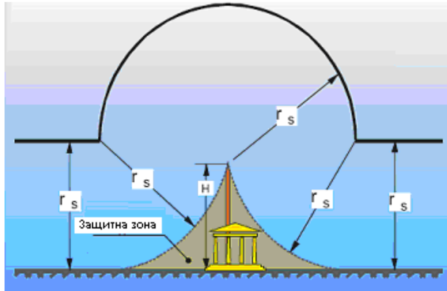
Фиг.1. Метод на въртящата се сфера (Електрогеометричен модел)
