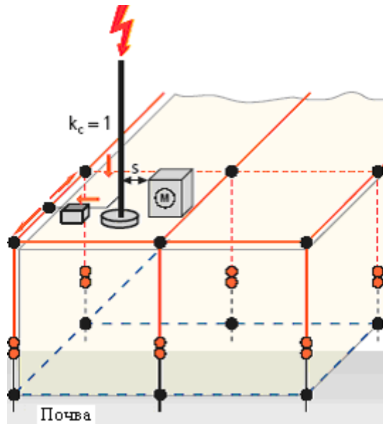
Фиг. 20. Плосък покрив с мълниеприемник прът и отдушник
